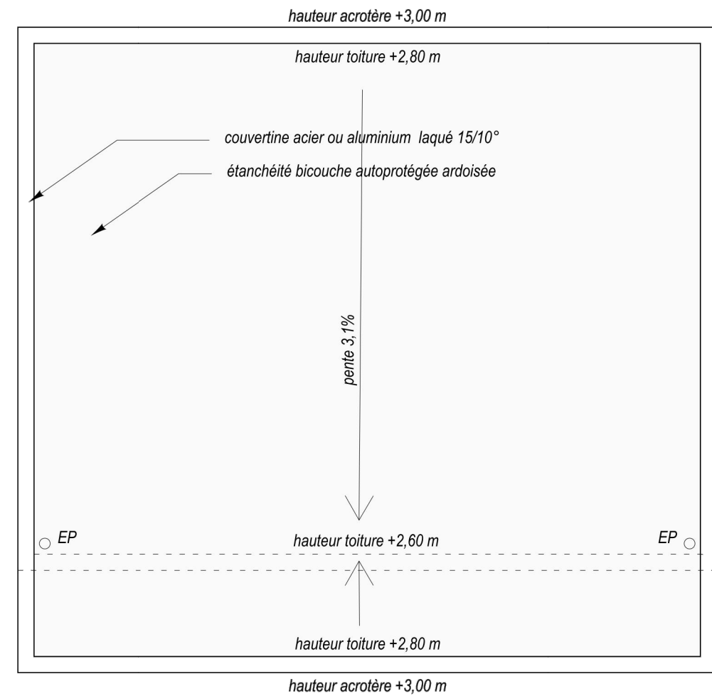
vue du plan de toiture
